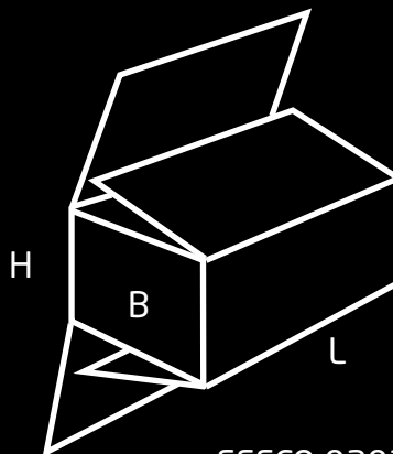
FEFCO 0203
