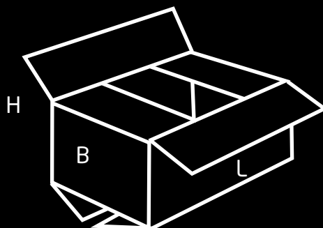
FEFCO 0201
